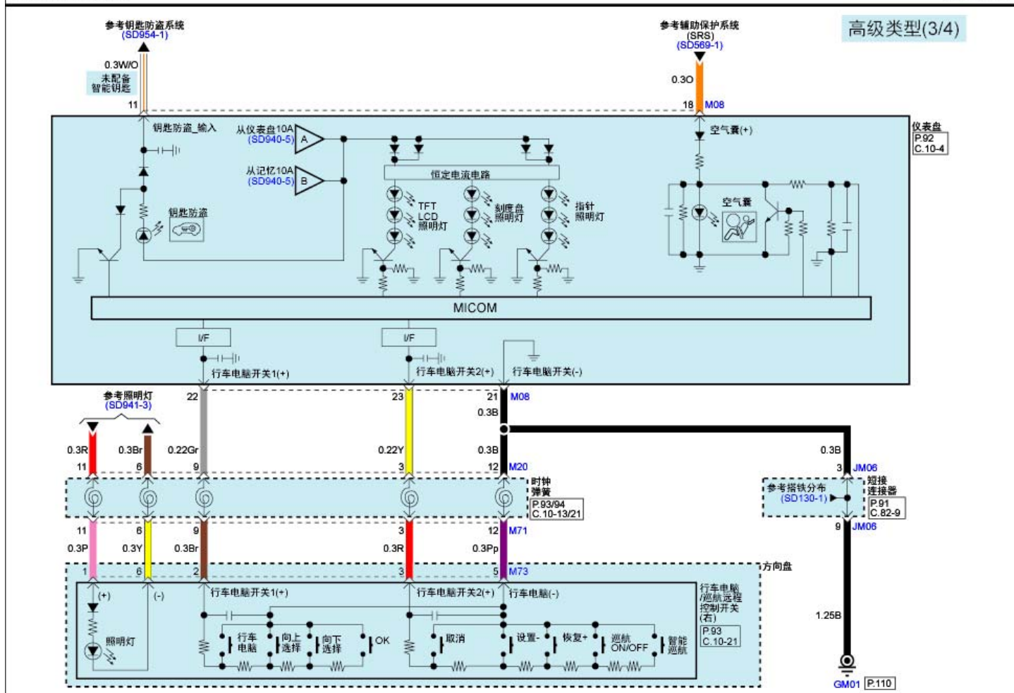
指示灯&amp;仪表(7)
